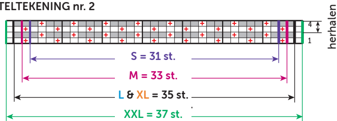
TELTEKENING nr. 2
